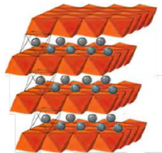
Estructura cristalina de NCA.
