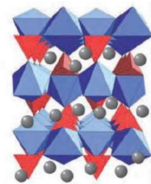
Estructura cristalina de LFP.
