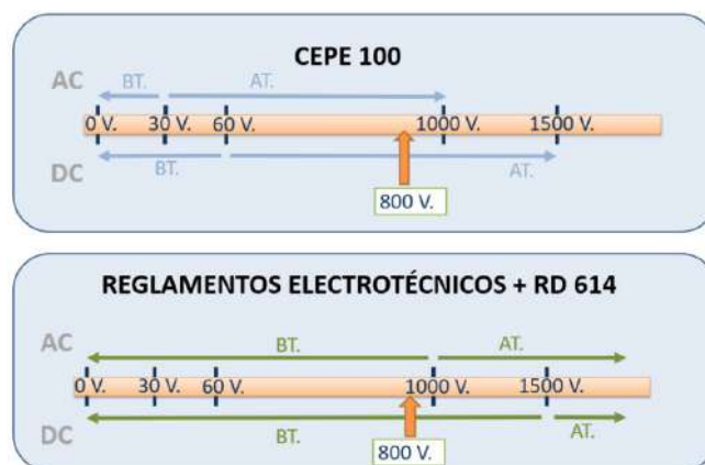
Comparativa entre AT vehicular y AT industrial (Fuente: SGS)
